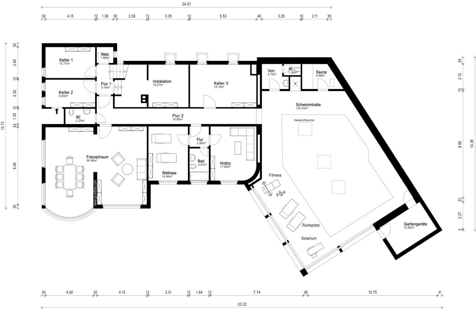
Kellergeschoss
